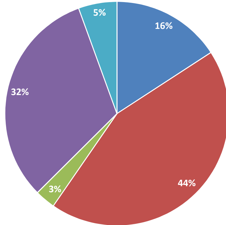
Structure des recettes d'investissement au BP 2023
